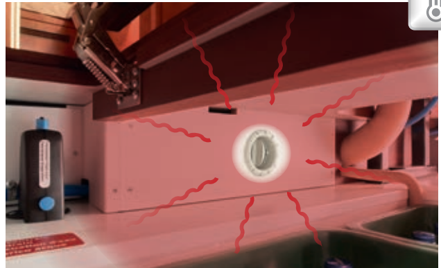
Wärmeluftspeicher-Heiztechnik Truma Combi 6 mit zahlreichen Wärmeluftauslässen im gesamten Doppelboden-Keller, im Wohnraum, in der Rollergarage und in den kältesensiblen Türeintriegen
